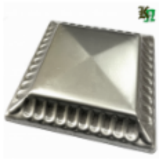
Основание баясины штампованное, арт. 8.880 170x170x1 Вес: 0.27 кг Цена: 135 руб.
