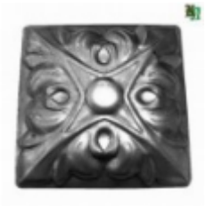
Накладка стальная, штампованная, арт. 8.849 100x100x1,2мм Вес: 0.08 кг Цена: 35 руб.
